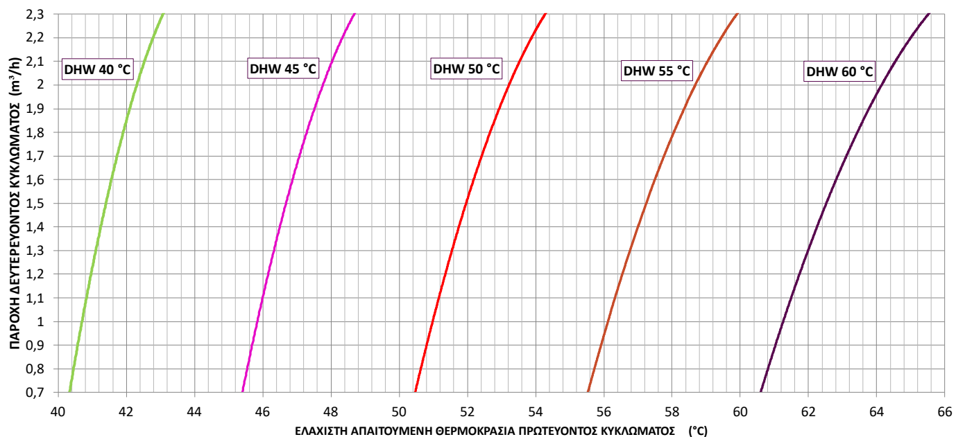
ΔΙΑΓΡΑΜΜΑ ΠΑΡΟΧΗΣ ΘΕΡΜΟΚΡΑΣΙΑΣ GSE CASCADE HE FW-CF 1/2
