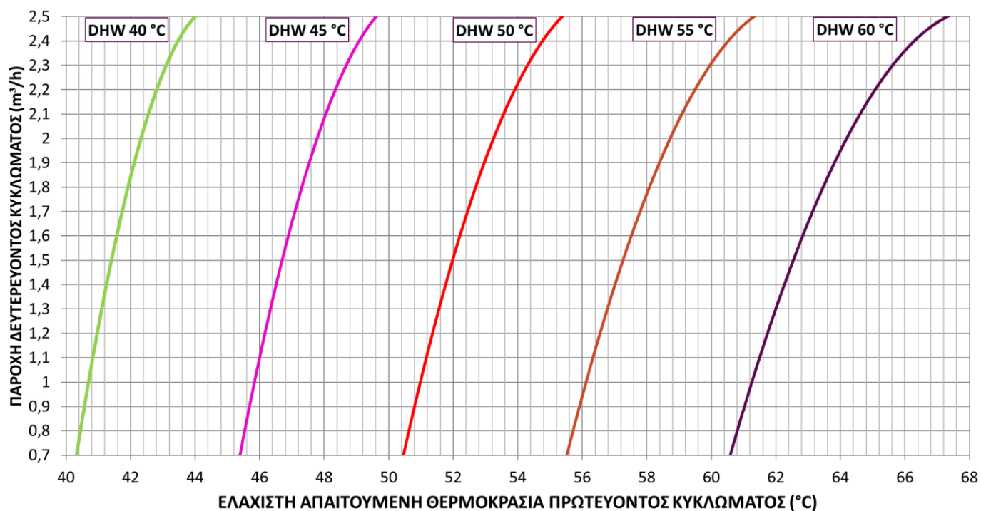
ΔΙΑΓΡΑΜΜΑ ΠΑΡΟΧΗΣ ΘΕΡΜΟΚΡΑΣΙΑΣ GSE CASCADE HE FW-CF 1/2
