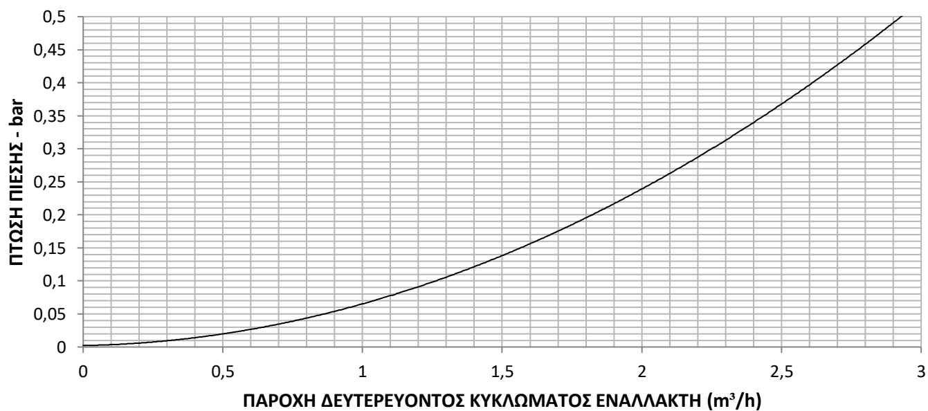
ΔΙΑΓΡΑΜΜΑ ΠΤΩΣΗΣ ΠΙΕΣΗΣ GSE CASCADE HE FW-CF 1/2 INOX/LR
