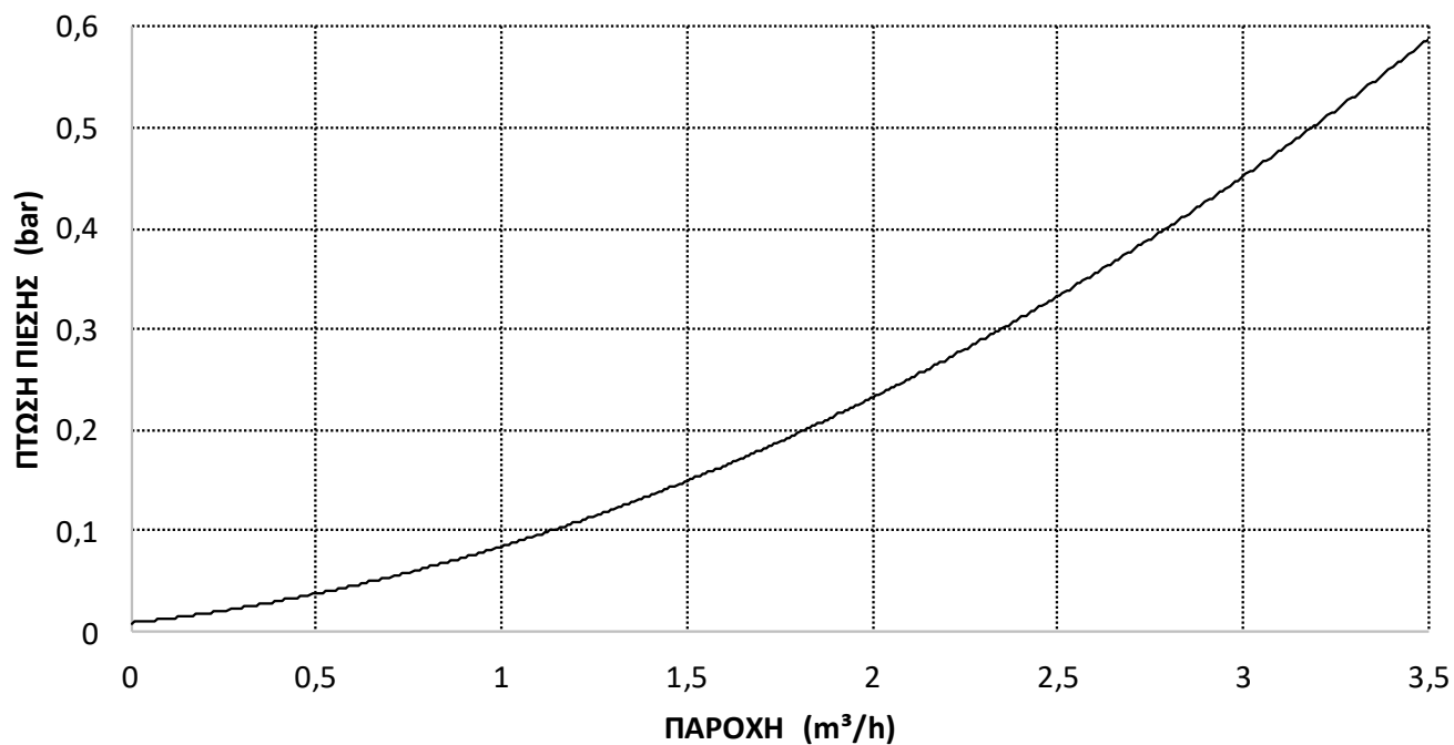
ΔΙΑΓΡΑΜΜΑ ΠΤΩΣΗΣ ΠΙΕΣΗΣ - ΠΑΡΟΧΗΣ GSE CASCADE BF VER-FW-F-S 1000
