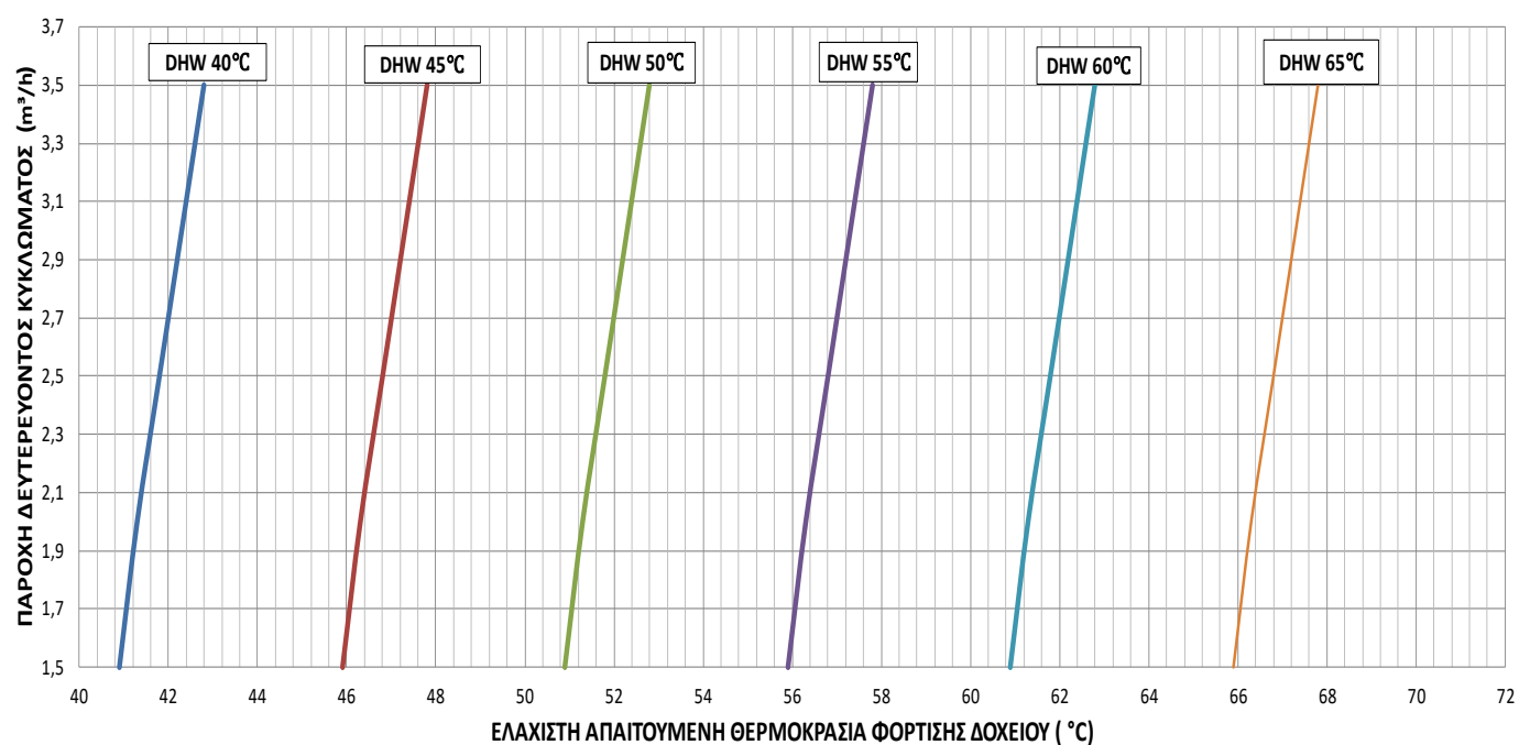
ΔΙΑΓΡΑΜΜΑ ΠΑΡΟΧΗΣ-ΘΕΡΜΟΚΡΑΣΙΑΣ GSE CASCADE BF VER-FW-F-S 1000
