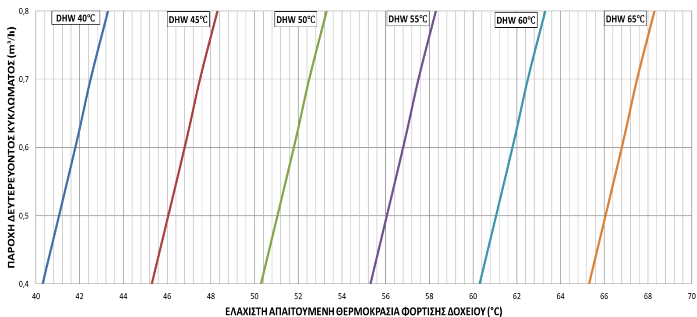
ΔΙΑΓΡΑΜΜΑ ΠΑΡΟΧΗΣ-ΘΕΡΜΟΚΡΑΣΙΑΣ GSE CASCADE BF VER-FW-F-S 150
