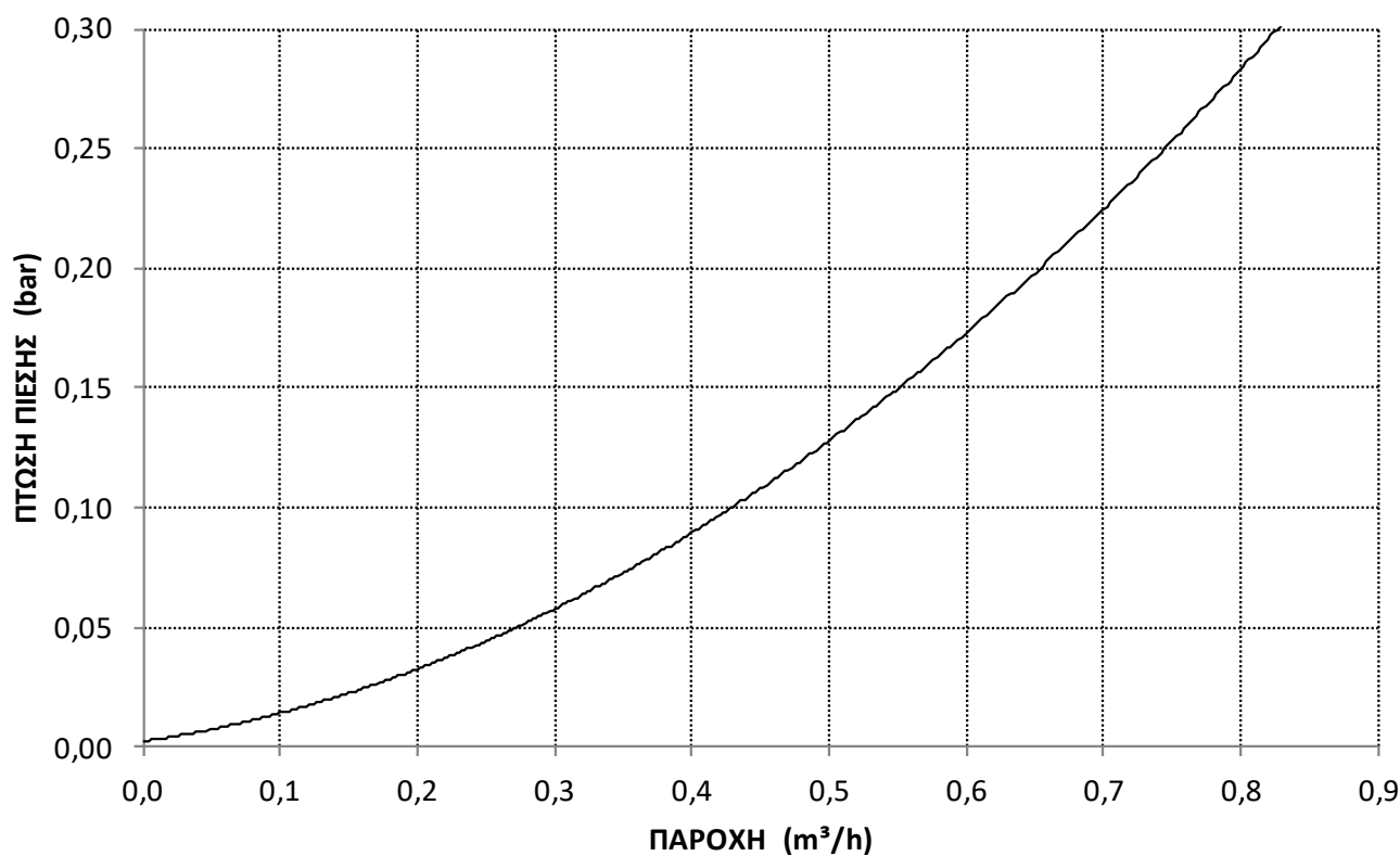
ΔΙΑΓΡΑΜΜΑ ΠΑΡΟΧΗΣ-ΘΕΡΜΟΚΡΑΣΙΑΣ GSE CASCADE BF VER-FW-F-S 150
