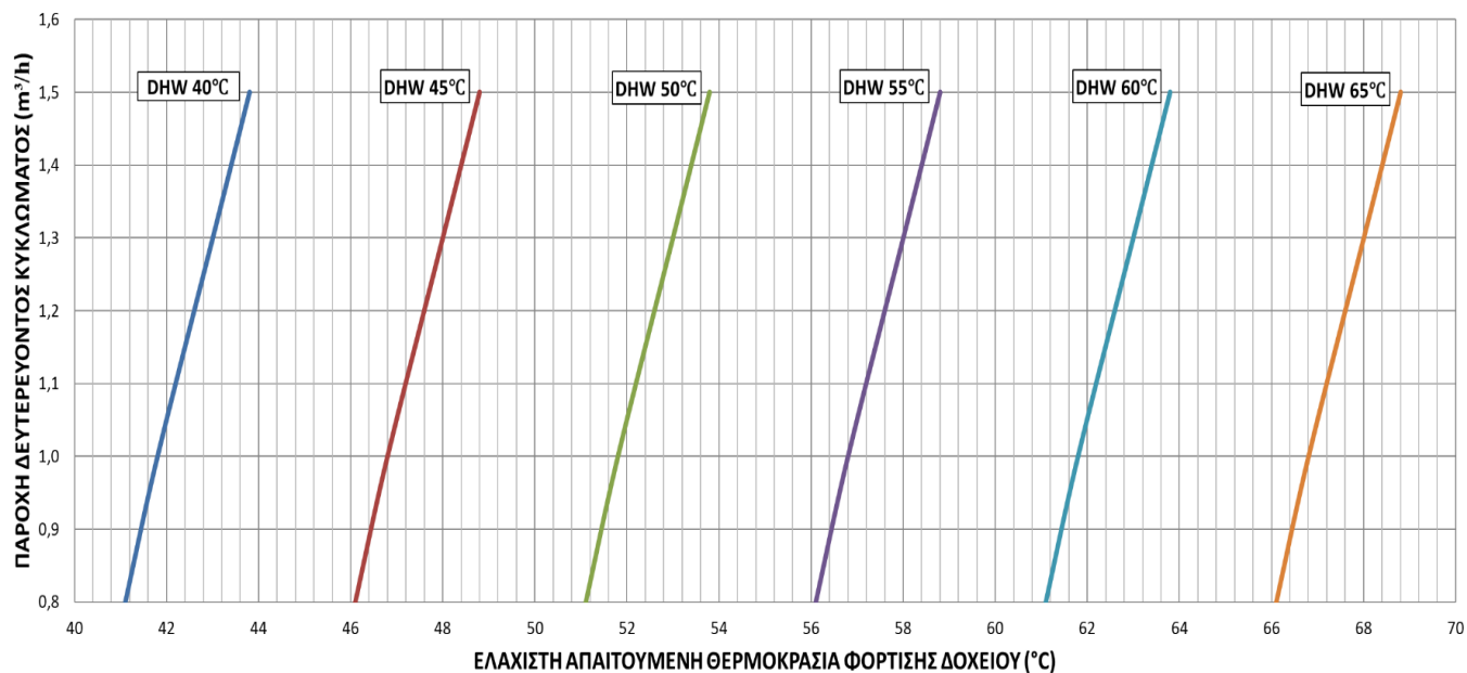
ΔΙΑΓΡΑΜΜΑ ΠΑΡΟΧΗΣ-ΘΕΡΜΟΚΡΑΣΙΑΣ GSE CASCADE BF VER-FW-F-S 200
