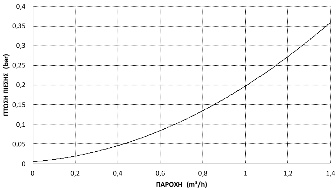
ΔΙΑΓΡΑΜΜΑ ΠΑΡΟΧΗΣ-ΘΕΡΜΟΚΡΑΣΙΑΣ GSE CASCADE BF-VER-F-S 200
