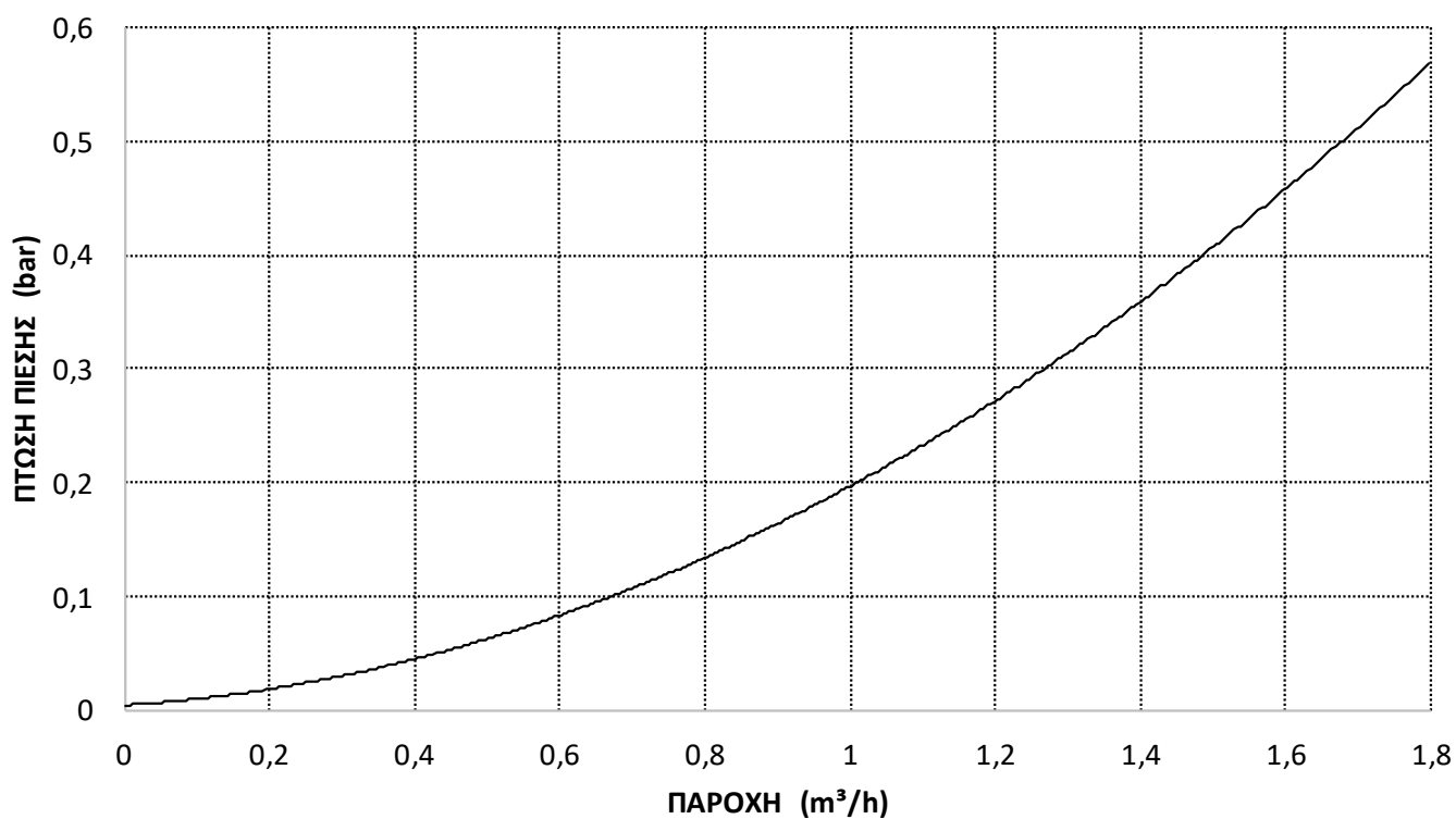
ΔΙΑΓΡΑΜΜΑ ΠΤΩΣΗΣ ΠΙΕΣΗΣ-ΠΑΡΟΧΗΣ GSE CASCADE BF VER-FW-F-S 300
