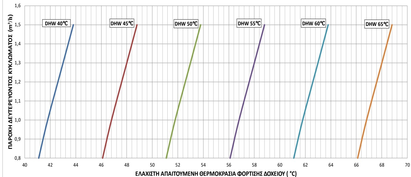
ΔΙΑΓΡΑΜΜΑ ΠΑΡΟΧΗΣ-ΘΕΡΜΟΚΡΑΣΙΑΣ GSE CASCADE BF VER-FW-F-S 300
