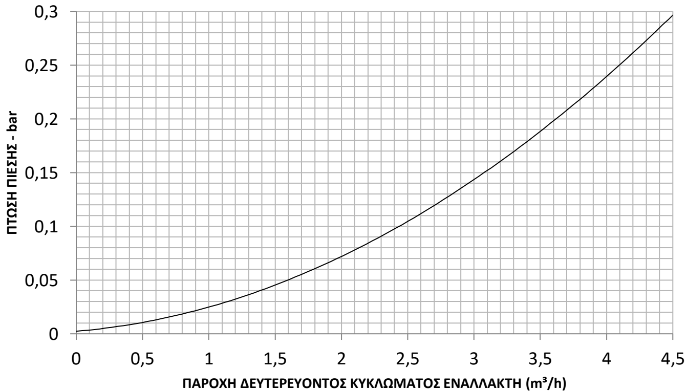
ΔΙΑΓΡΑΜΜΑ ΠΤΩΣΗΣ ΠΙΕΣΗΣ GSE CASCADA HE FW-CF 1/3 INOX/LR
