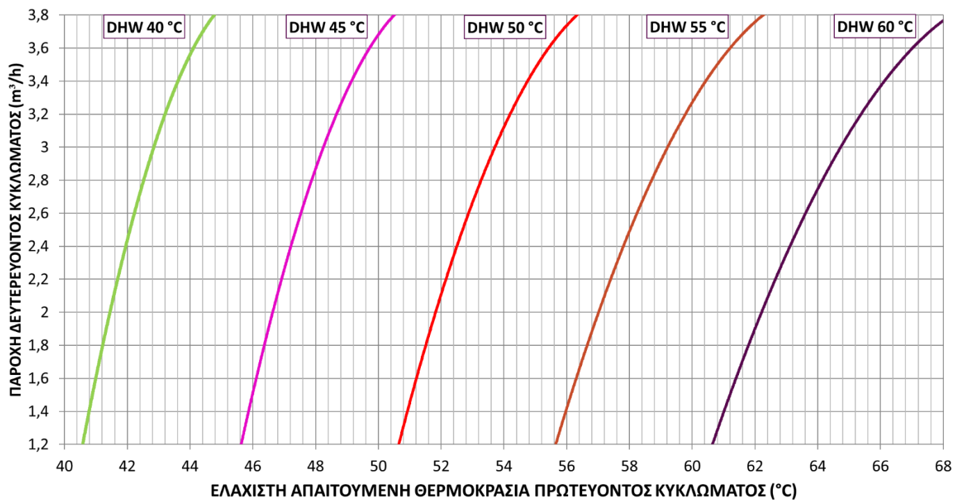
ΔΙΑΓΡΑΜΜΑ ΠΑΡΟΧΗΣ ΘΕΡΜΟΚΡΑΣΙΑΣ GSE CASCADE HE FW-CF 1/3
