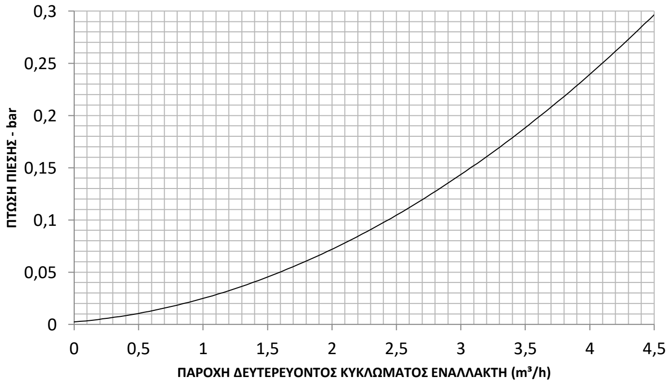
ΔΙΑΓΡΑΜΜΑ ΠΤΩΣΗΣ ΠΙΕΣΗΣ GSE CASCADE HE FW-CF 1/3 INOX/LR
