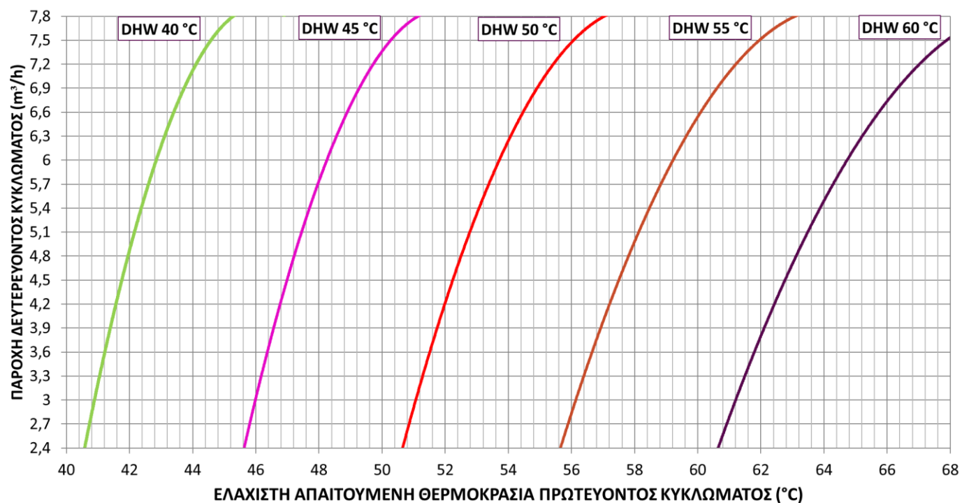
ΔΙΑΓΡΑΜΜΑ ΠΑΡΟΧΗΣ ΘΕΡΜΟΚΡΑΣΙΑΣ GSE CASCADE HE FW-CF 2/3
