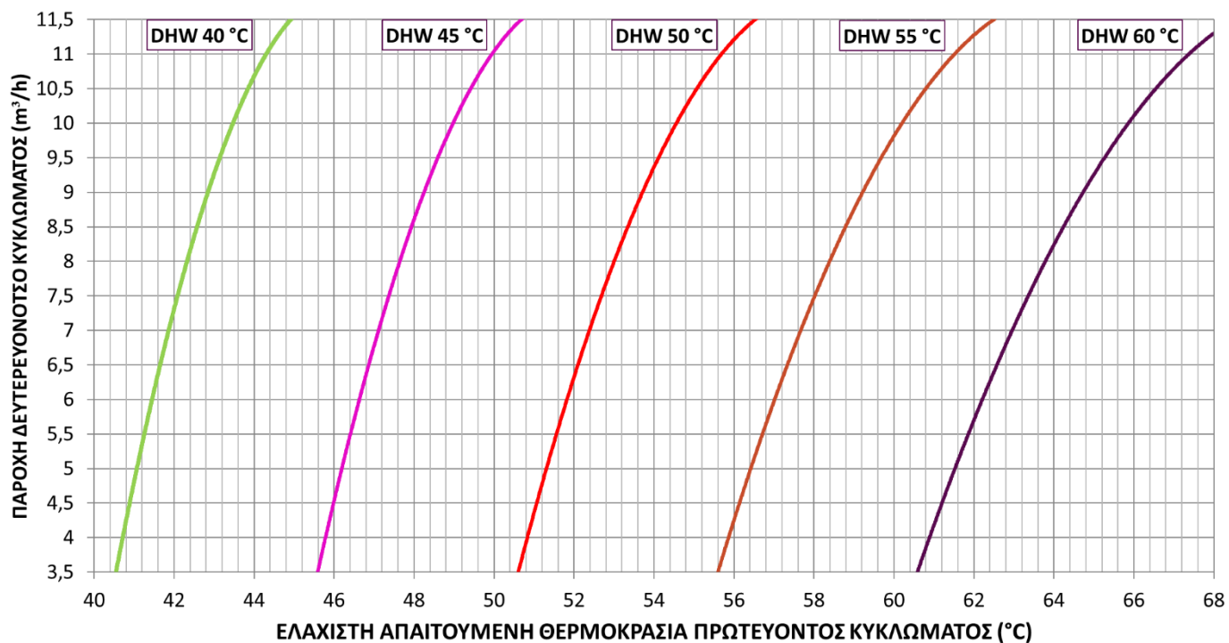
ΔΙΑΓΡΑΜΜΑ ΠΑΡΟΧΗΣ ΘΕΡΜΟΚΡΑΣΙΑΣ GSE CASCADE HE FW-CF 3/3
