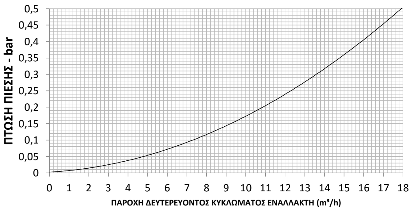
ΔΙΑΓΡΑΜΜΑ ΠΤΩΣΗΣ ΠΙΕΣΗΣ GSE CASCADE HE FW-CF 3/3 INOX/LR
