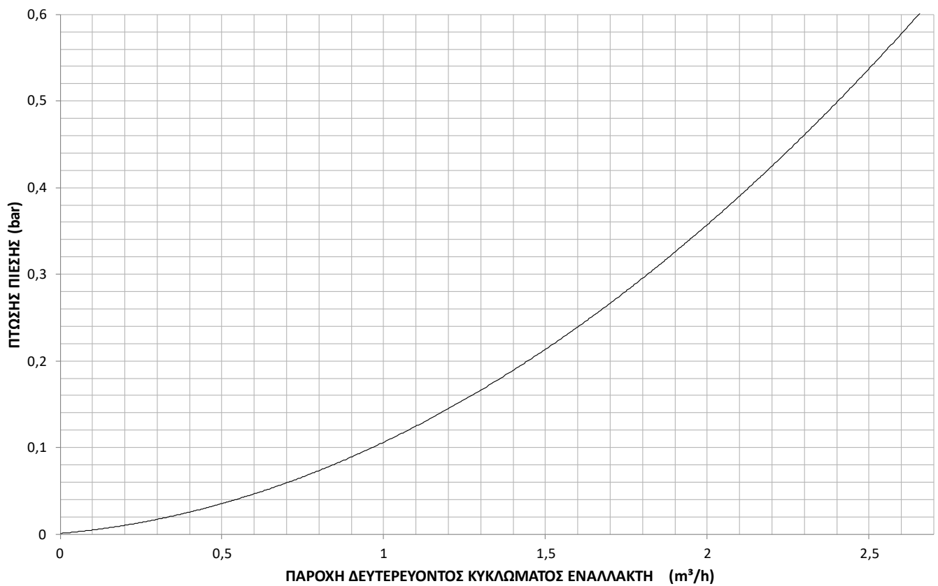
ΔΙΑΓΡΑΜΜΑ ΠΤΩΣΗΣ ΠΙΕΣΗΣ-ΠΑΡΟΧΗΣ GSE CASCADE BF VER-FW-CF-S 1000/20
