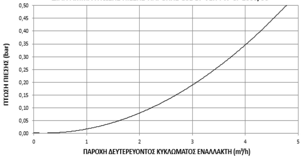
ΔΙΑΓΡΑΜΜΑ ΠΤΩΣΗΣ ΠΙΕΣΗΣ-ΠΑΡΟΧΗΣ GSE BF VER-FW-CF 1000/30
