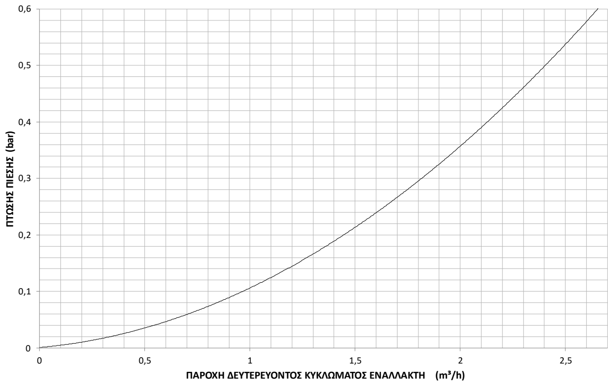
ΔΙΑΓΡΑΜΜΑ ΠΤΩΣΗΣ ΠΙΕΣΗΣ-ΠΑΡΟΧΗΣ GSE CASCADE BF VER-FW-CF 1000/20
