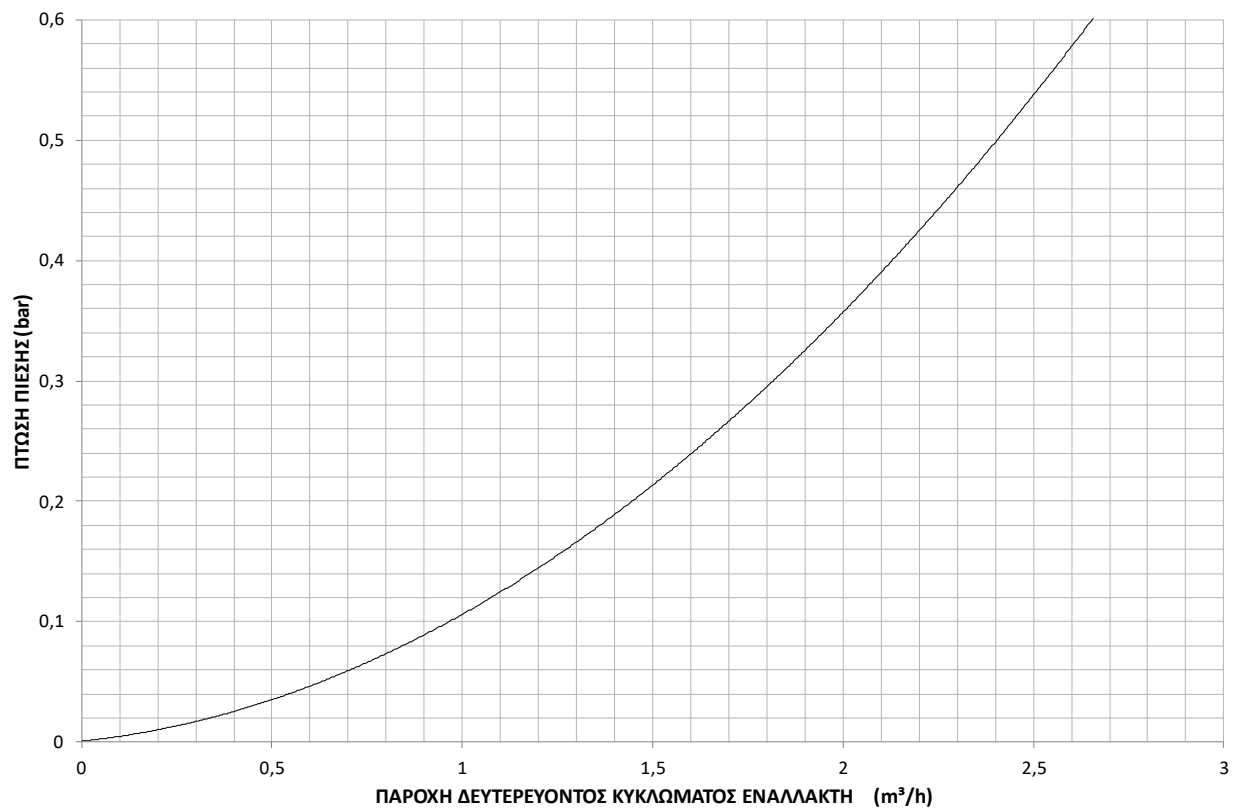
ΔΙΑΓΡΑΜΜΑ ΠΤΩΣΗΣ ΠΙΕΣΗΣ-ΠΑΡΟΧΗΣ GSE CASCADE BF VER-FW-CF 600/20
