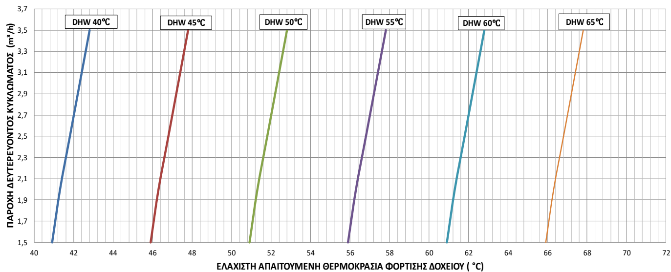
ΔΙΑΓΡΑΜΜΑ ΠΑΡΟΧΗΣ-ΘΕΡΜΟΚΡΑΣΙΑΣ GSE CASCADE BF VER-FW-F 1000
