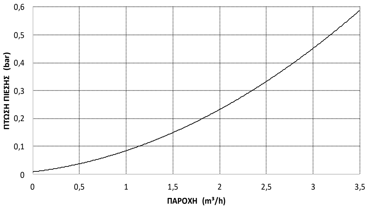
ΔΙΑΓΡΑΜΜΑ ΠΤΩΣΗΣ ΠΙΕΣΗΣ-ΠΑΡΟΧΗΣ GSE CASCADE BF VER-FW-F 1000
