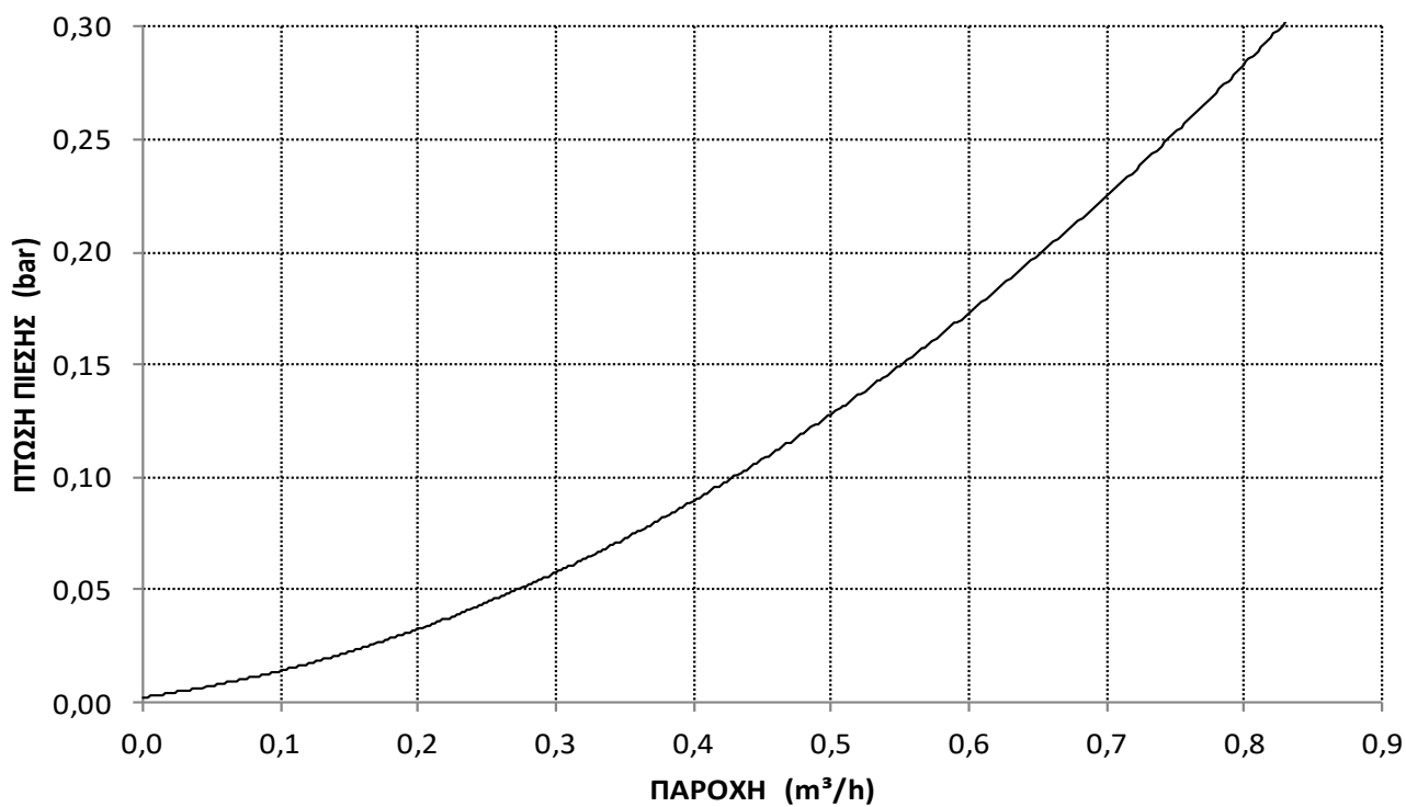
ΔΙΑΓΡΑΜΜΑ ΠΑΡΟΧΗΣ-ΘΕΡΜΟΚΡΑΣΙΑΣ GSE CASCADE BF VER-FW-F 150
