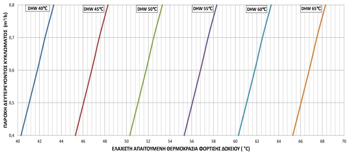
ΔΙΑΓΡΑΜΜΑ ΠΑΡΟΧΗΣ-ΘΕΡΜΟΚΡΑΣΙΑΣ GSE CASCADE BF VER-FW-F 150
