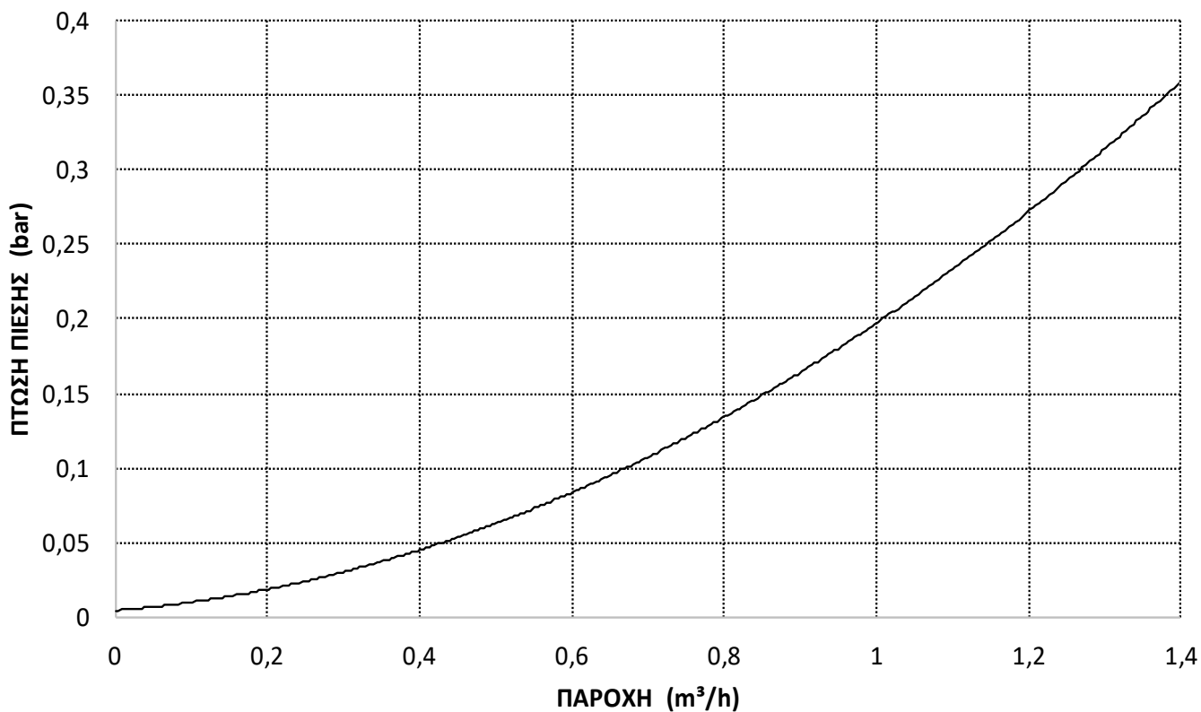
ΔΙΑΓΡΑΜΜΑ ΠΑΡΟΧΗΣ-ΘΕΡΜΟΚΡΑΣΙΑΣ GSE CASCADE BF-VER-F 200
