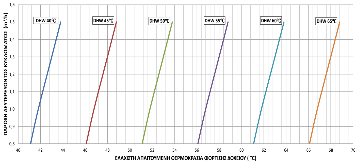
ΔΙΑΓΡΑΜΜΑ ΠΑΡΟΧΗΣ-ΘΕΡΜΟΚΡΑΣΙΑΣ GSE CASCADE BF VER-FW-F 200
