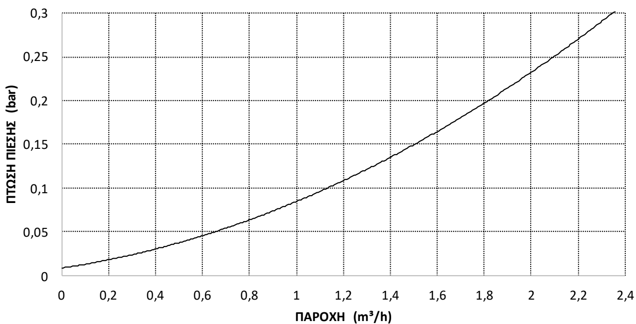
ΔΙΑΓΡΑΜΜΑ ΠΤΩΣΗΣ ΠΙΕΣΗΣ-ΠΑΡΟΧΗΣ GSE CASCADA BF VER-FW-F 600
