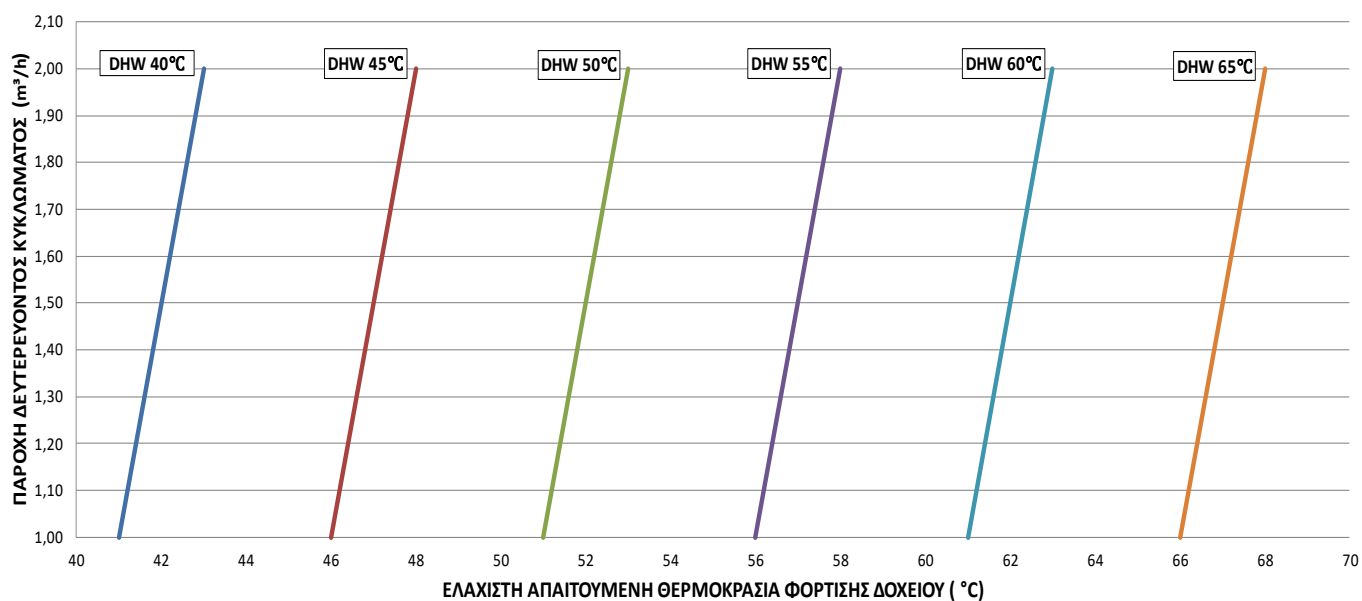
ΔΙΑΓΡΑΜΜΑ ΠΑΡΟΧΗΣ-ΘΕΡΜΟΚΡΑΣΙΑΣ GSE CASCADA BF VER-FW-F 600
